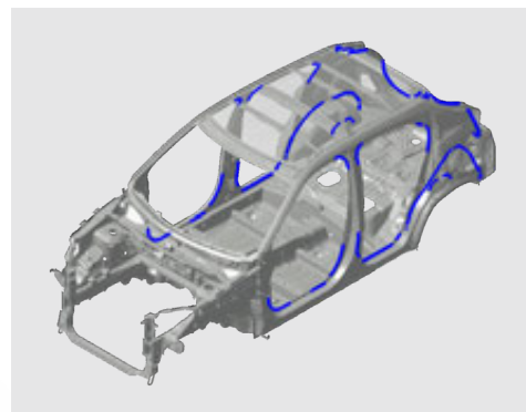
Използваните структурни адхезиви в отворите на страничните врати и задната врата укрепват връзката между отделните части. (Илюстрациите са дадени само с цел онагледяване.)
